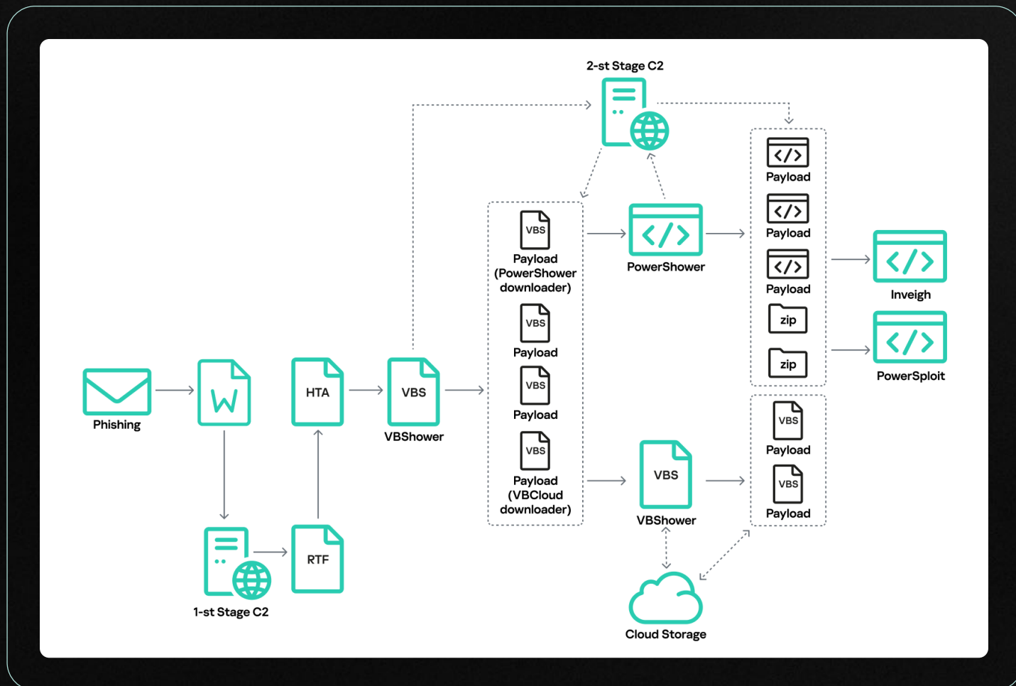
Рис. 43 | Типовая схема заражения Cloud Atlas
